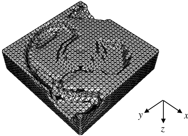
誘電体の最適構造
