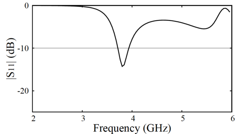
反射特性(初期構造)
