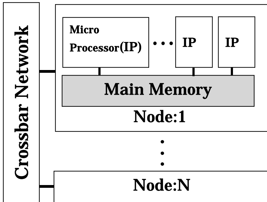
スーパーコンピュータ SR8000 の構造図
